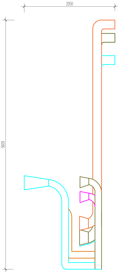
MẶT ĐÚNG BÊN NHÓM ỐNG 1
