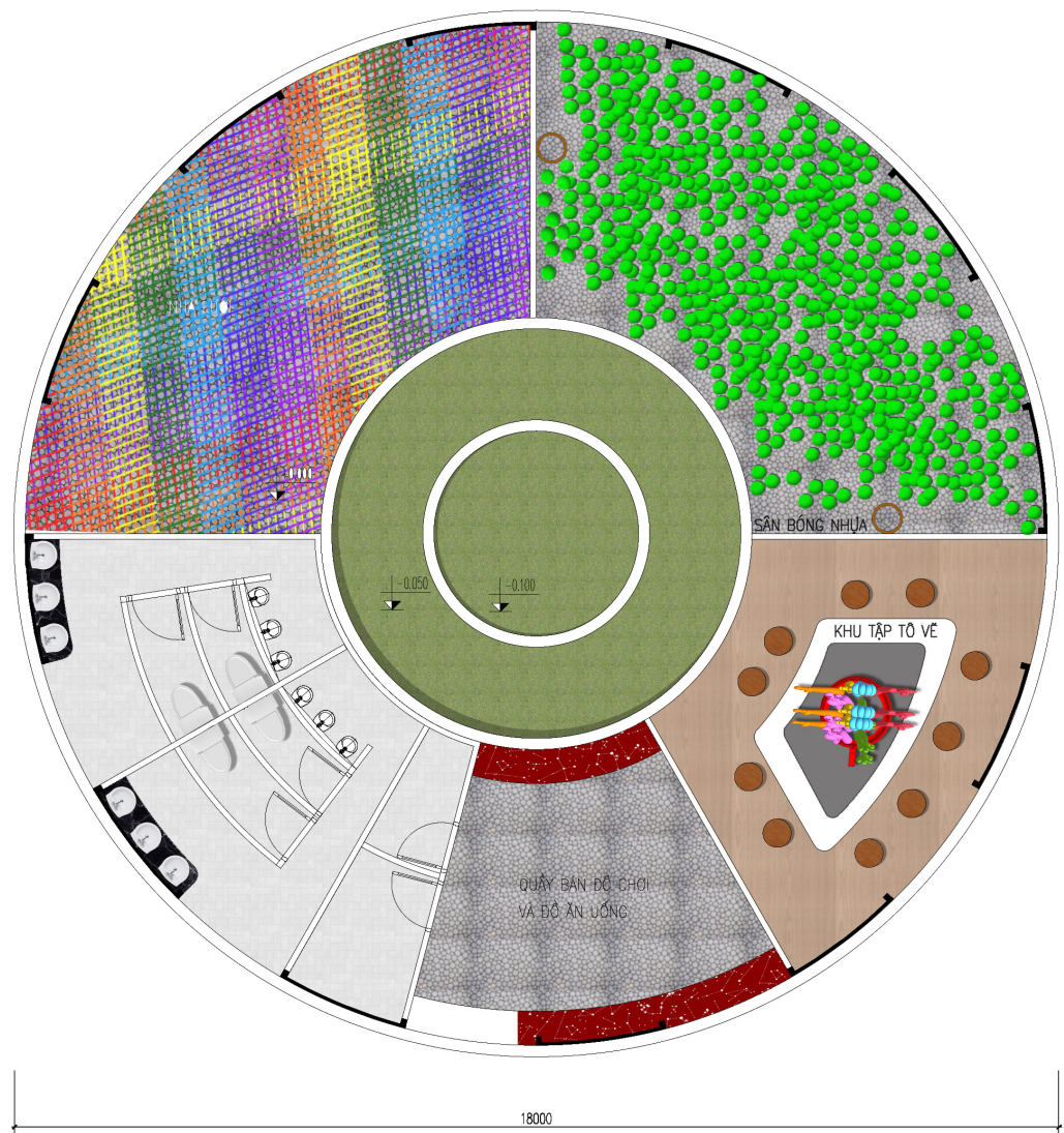
MẶT BẰNG
