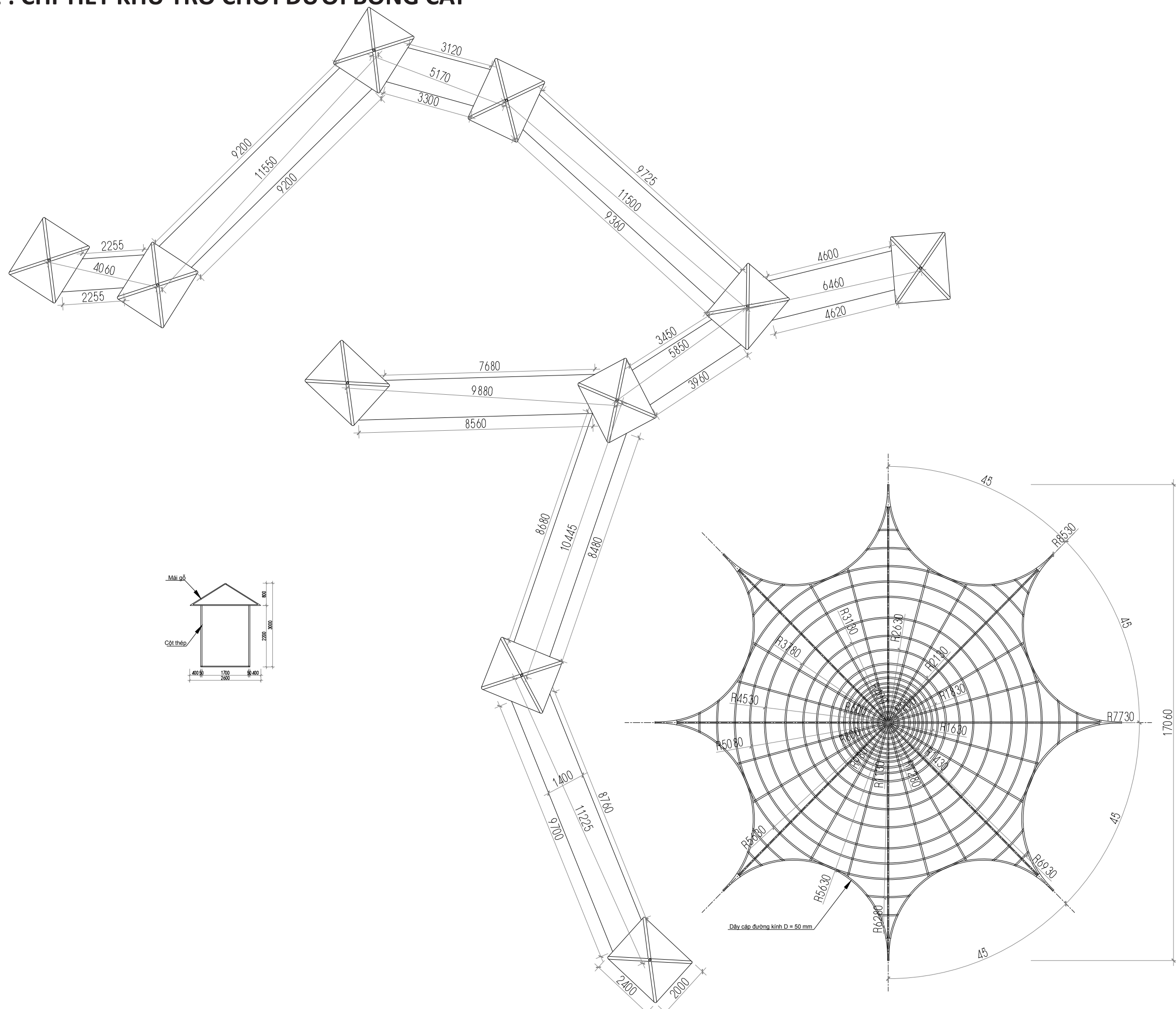
IMAGE 25.2 : CHI TIẾT KHU TRÒ CHƠI DƯỚI BÓNG CÂY
