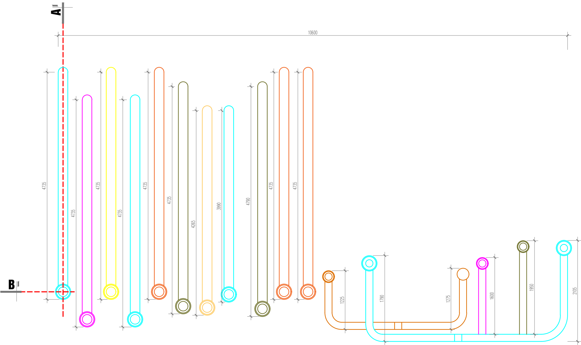
IMAGE 15.3: CHI TIẾT KÍCH THƯỚC ỐNG NGHE
